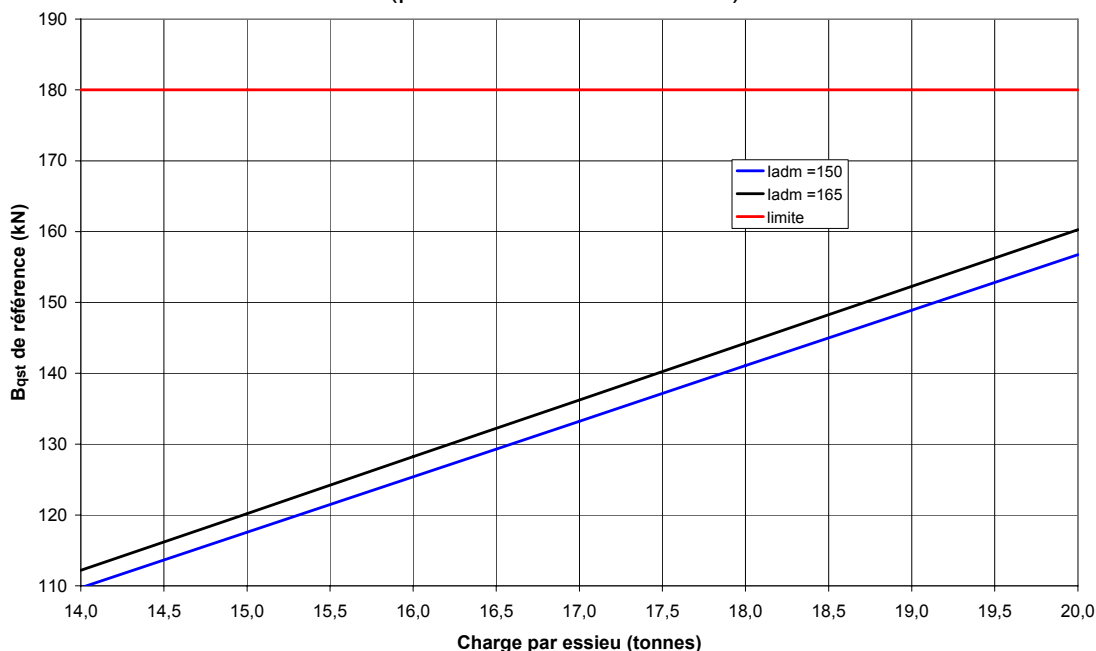
Evaluation théorique de B_{qst} pour les automotrices (pour R = 350 \text{ m} et I = I_{adm} )
